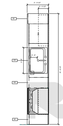
Details Plan - Comptoir Est
