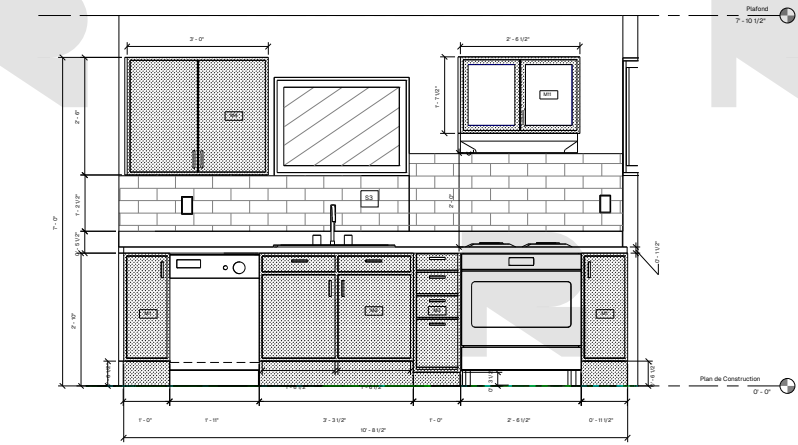
③ Elévation Cuisine - Est
